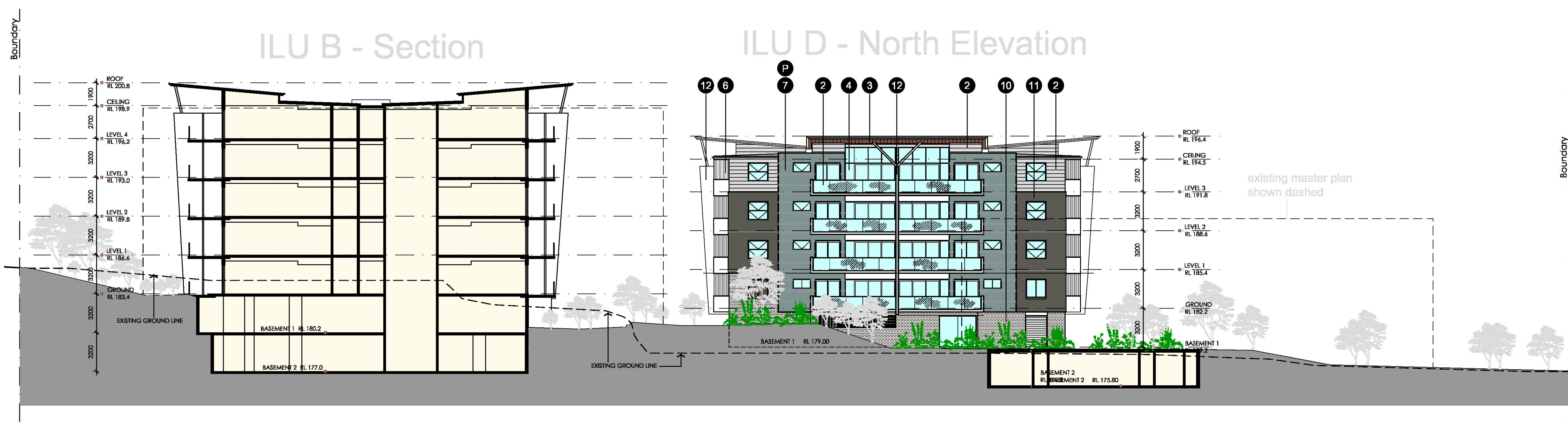
SITE SECTION 4
