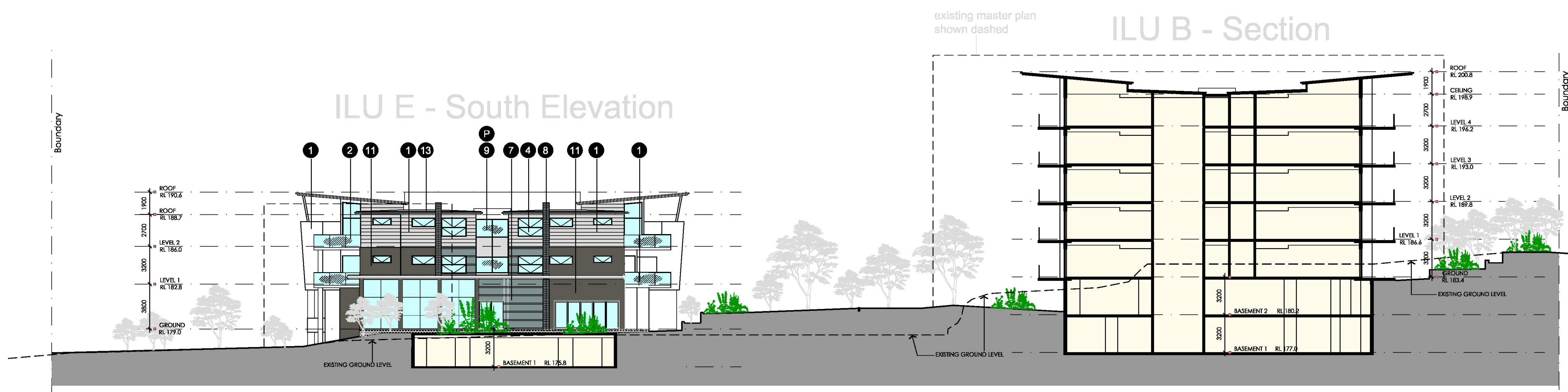
SITE SECTION 2
